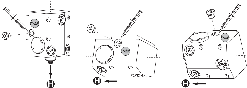
图片 19： 加注器螺钉的位置取决于安装方向。示例：U 版本
