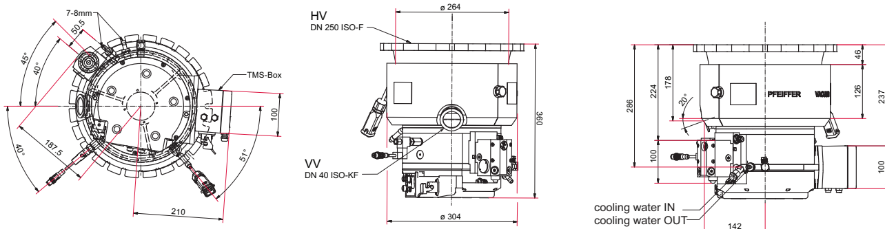
图片 36: HiPace 1500 T | TC 1200 DN 250 ISO-F
