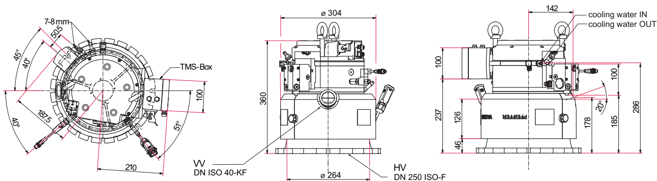
图片 38: HiPace 1500 UT | TC 1200 DN 250 ISO-F
