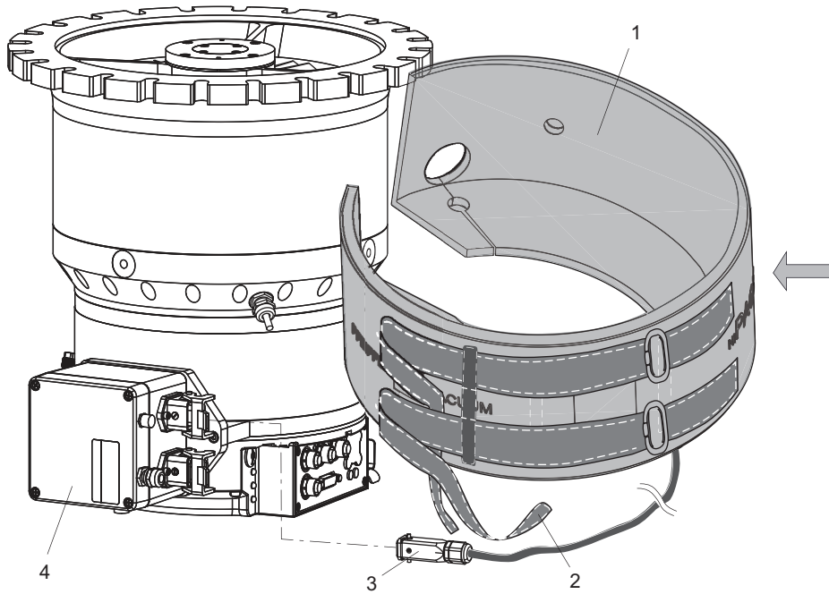
图片 31: 装配加热套
