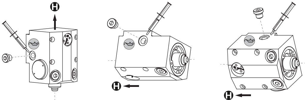
图片 26： 加注器螺钉的位置取决于安装方向。示例：标准版本
