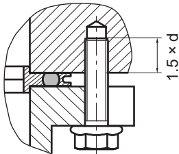
图片 15: 法兰连接 ISO-F, 六角头螺钉和螺纹孔
