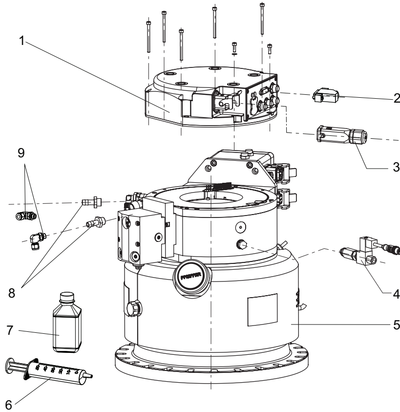
图片 34: HiPace 1500 T | UT 的备件
