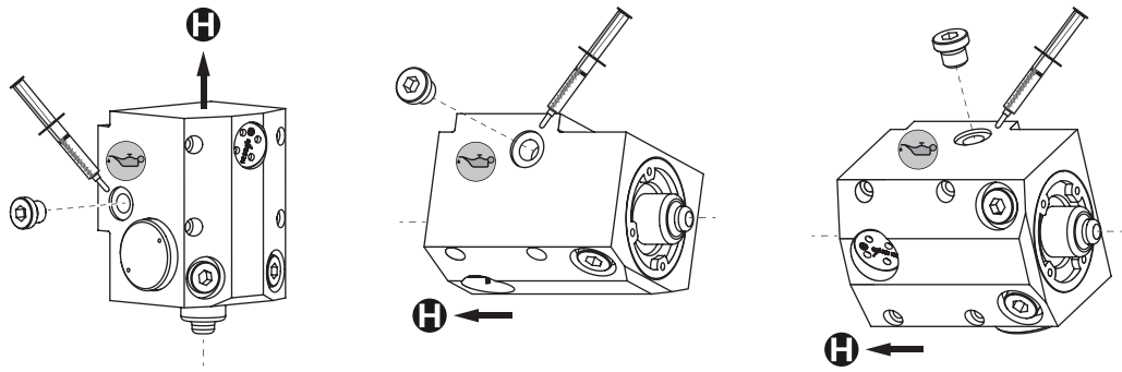
图片 18： 加注器螺钉的位置取决于安装方向。示例：标准版本
