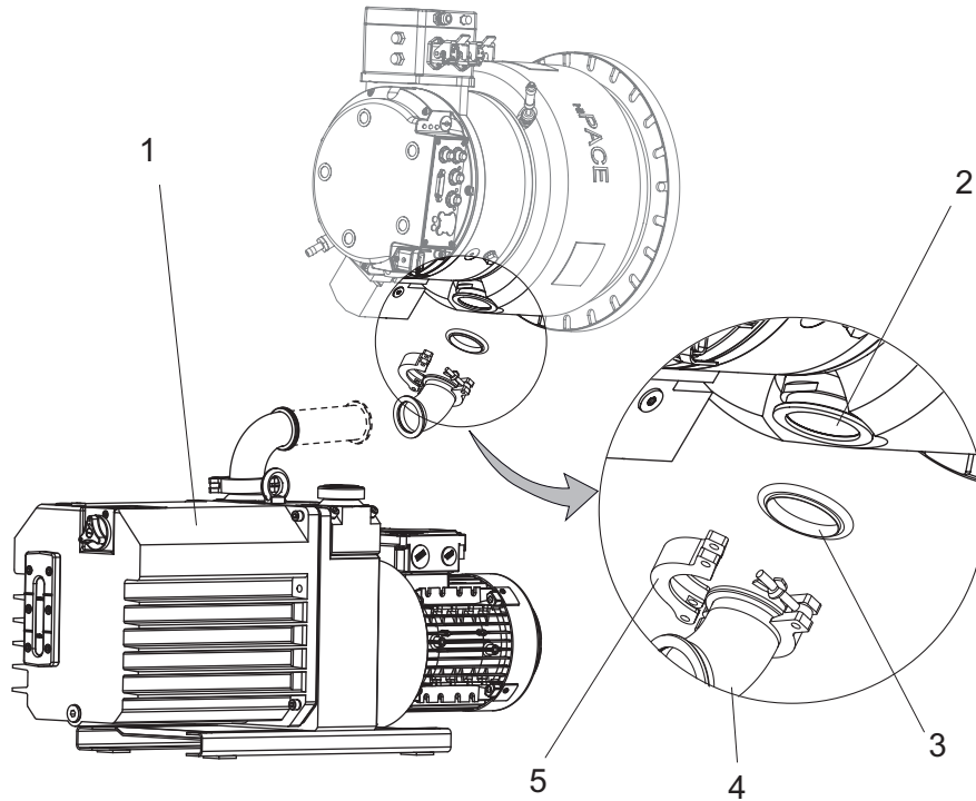
图片 20: HiPace 1500 T 的前级真空连接
