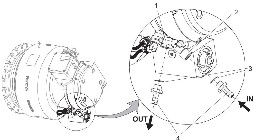
图片 21: 将冷却水连接装置连接到软管嘴上
