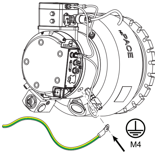
图片 23: 示例:连接接地电缆
