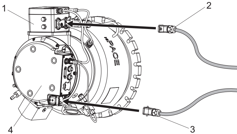
图片 24: HiPace 1500 T | UT 电源连接
