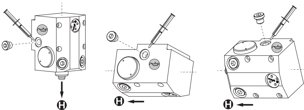
图片 27： 加注器螺钉的位置取决于安装方向。示例：U 版本
