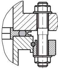
图片 14: ISO-K 到 ISO-F 的法兰连接、螺栓和通孔
