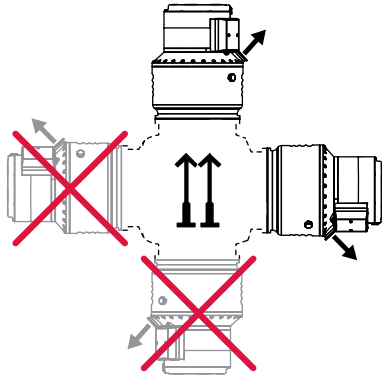
图片 9： U 型涡轮泵的安装方向(架空)
