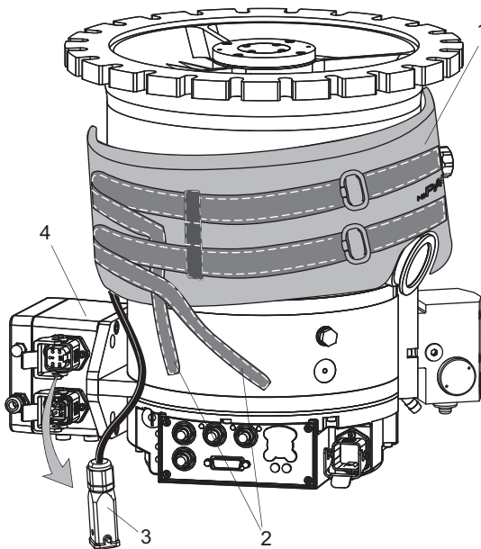
图片 30: 拆卸加热套
