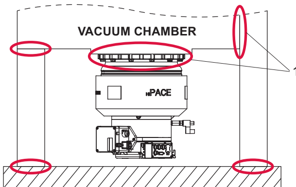
图片 7: 示例: 固定好以防止外部振动引起的位移和倾斜
