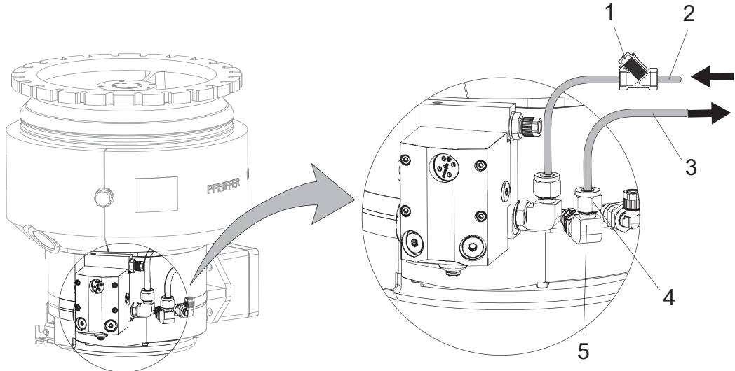
图片 22: 将冷却水连接装置连接到管道接头上
