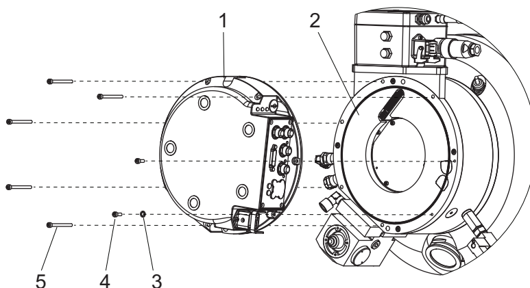
图片 28： 拆卸电子驱动单元
