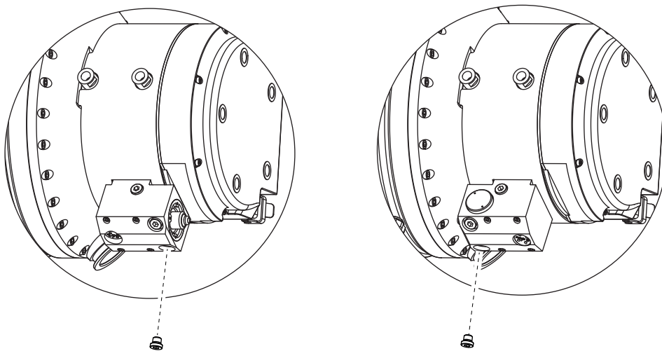
图片 25: 示例:标准型号和 U 型涡轮泵上工作液的排放方法
