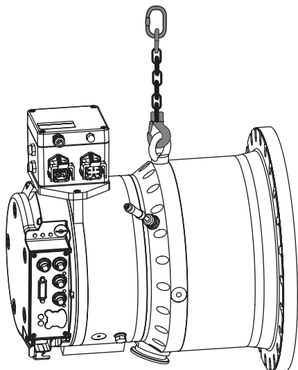
图片 6： 未包装的涡轮泵水平运输的吊点
