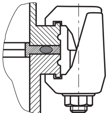
图片 11： ISO-K 至 ISO-F 的法兰连接, 支架螺钉
