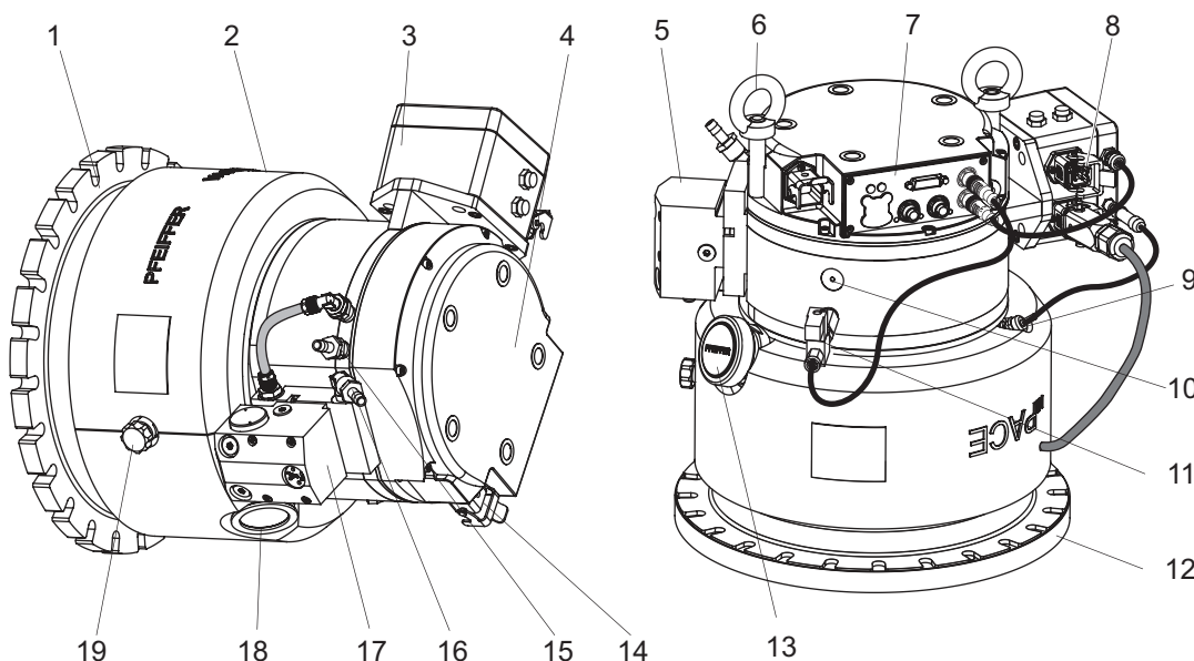
图片 3: HiPace 1500 T | UT 设计
