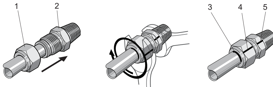
图片 33: 安装管道接头
