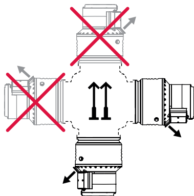
图片 8: 标准版安装方向(落地式)
