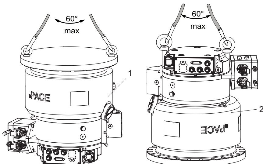
图片 5： 拆箱后垂直运输涡轮泵的起吊点
