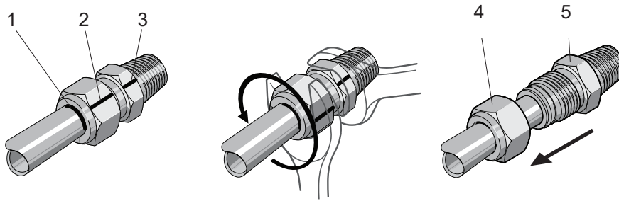
图片 32: 拆卸管道接头
