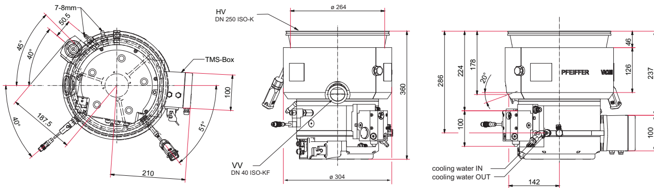
图片 35: HiPace 1500 T | TC 1200 DN 250 ISO-K
