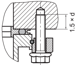
图片 12: ISO-K 到 ISO-F 的法兰连接、六角头螺钉和螺纹孔
