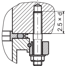
图片 13: ISO-K 到 ISO-F 的法兰连接、螺杆和螺纹孔
