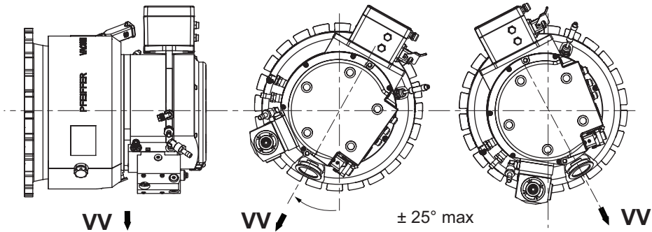
图片 10： 前置真空连接必须与水平安装方向一致
