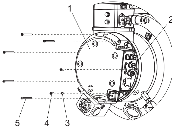
图片 29: 固定电子驱动单元
