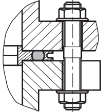
图片 17: ISO-F 法兰连接, 螺杆和通孔
