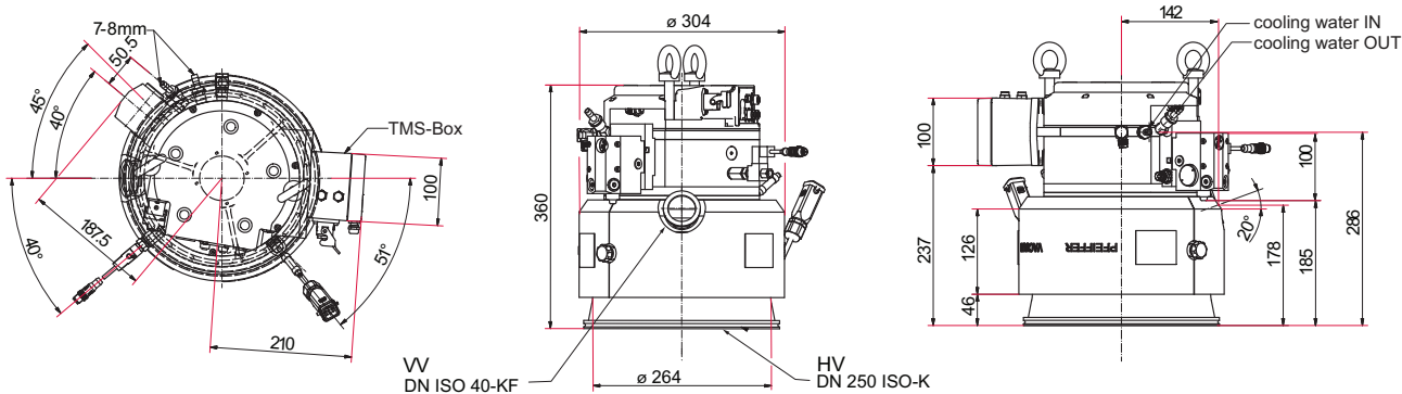
图片 37: HiPace 1500 UT | TC 1200 DN 250 ISO-K
