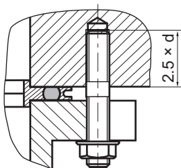
图片 16: 法兰连接 ISO-F, 螺栓和螺纹孔
