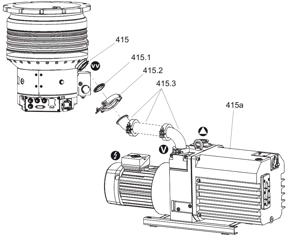
图 10: 连接前级泵
