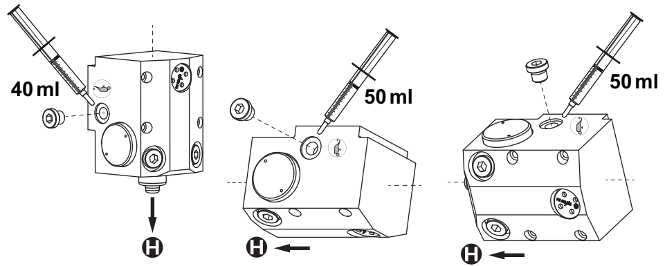
图 19: 在各自的有效空间位置给“U”型和“UC”型 HiPace 2300 添加工作流体
