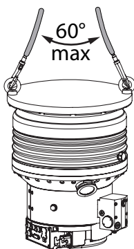
图 1: HiPace 2300 的运输
