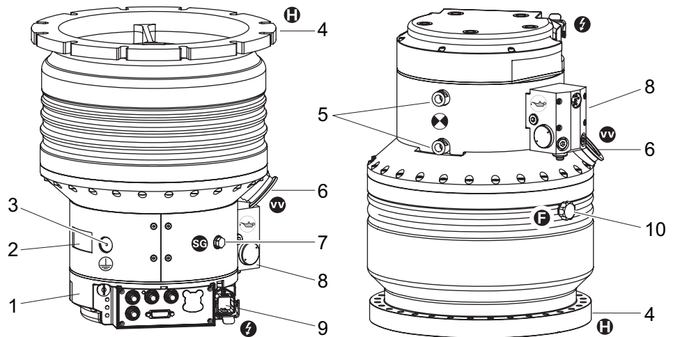
图 4: 带 TC 1200 的 HiPace 2300，标准型和“U”型
