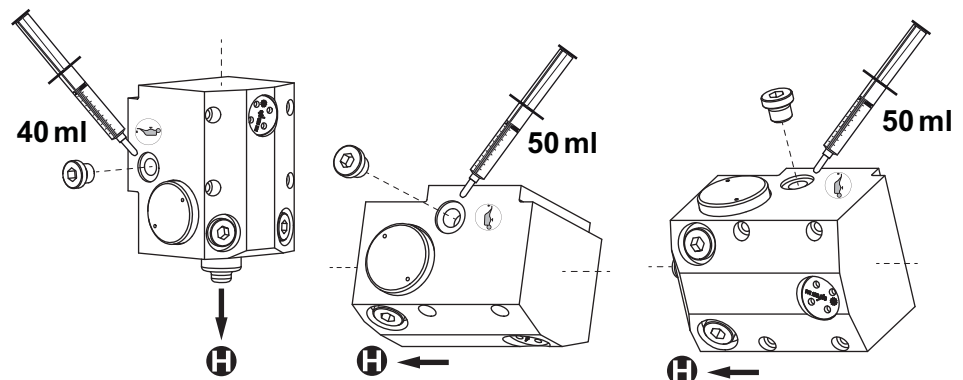
图 9: 在各自的有效空间位置给“U”型和“UC”型 HiPace 2300 添加工作流体
