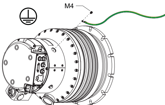
图 11: 建立接地连接
