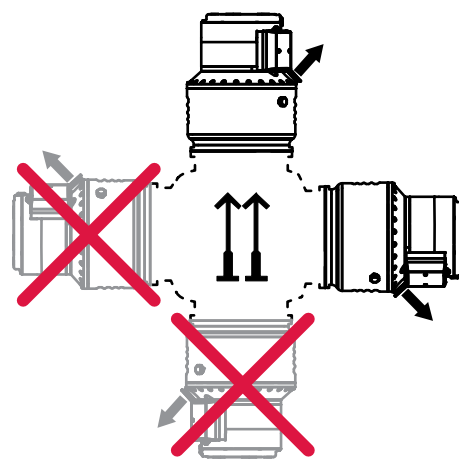
图 7: U 型和 UC 型
