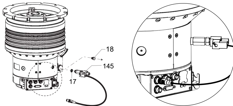
图 13: 连接气体吹扫阀
