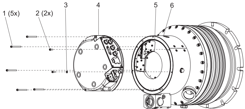
图 20: 拆卸 / 安装 TC 1200
