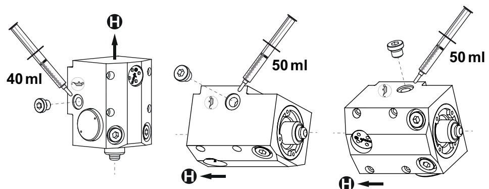
图 18: 在各自的有效空间位置给标准型和“C”型 HiPace 2300 添加工作流体
