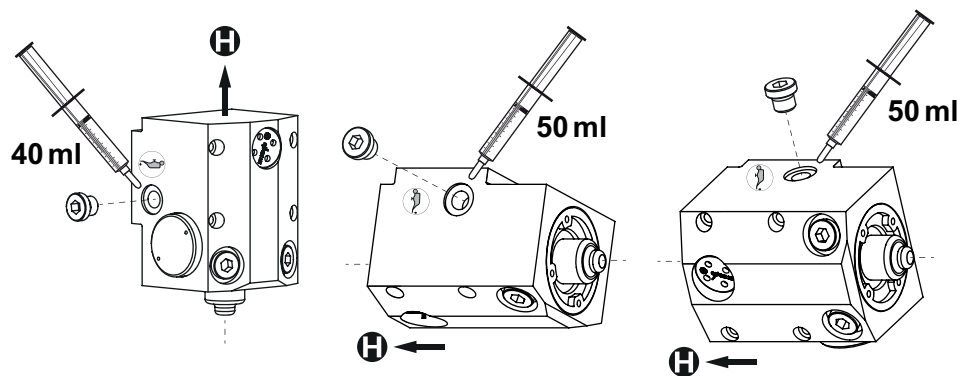
图 8: 在各自的有效空间位置给标准型和“C”型 HiPace 2300 添加工作流体
