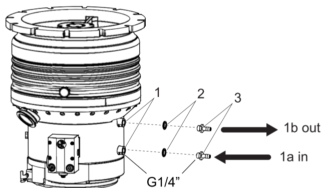
图 15: 连接冷却水
