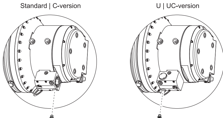
图 17: 在各自的水平安装位置为标准型和 U 型 HiPace 2300 添加工作流体
