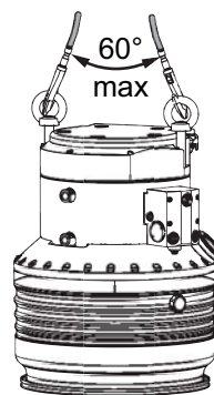
图 2: HiPace 2300 U 的运输
