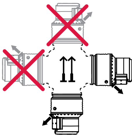
图 6: 标准型和 C 型
